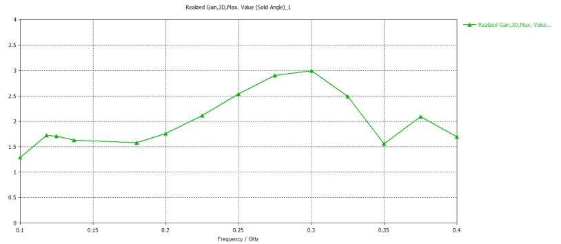
Frekansa Bağlı Anten Kazancı
