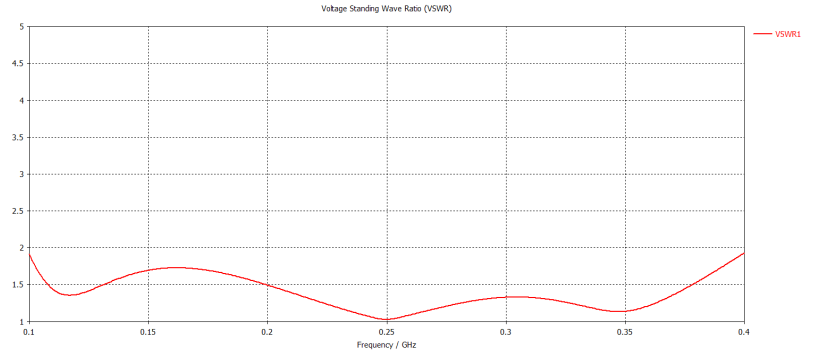
Frekansa Bağlı VSWR
