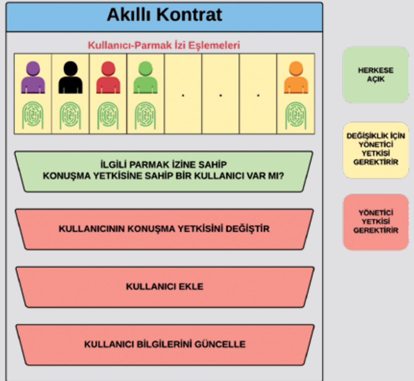
Şekil 3: Hazırlanan akıllı sözleşme
