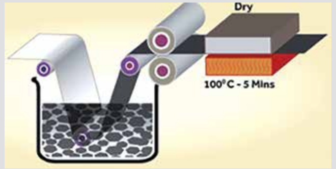
Grafen bazlı tekstil üretim şeması
